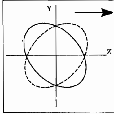
D- الحالة الثانية لاستقطاب الموجة التجاذبية الصريف
